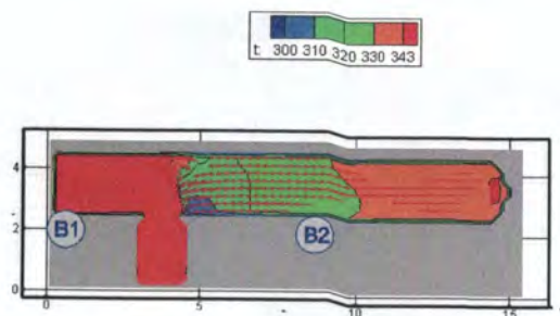
Рис. 165. Поля температуры (K) в горизонтальном сечении на высоте 1,7 м от уровня пола в момент времени 190 с
