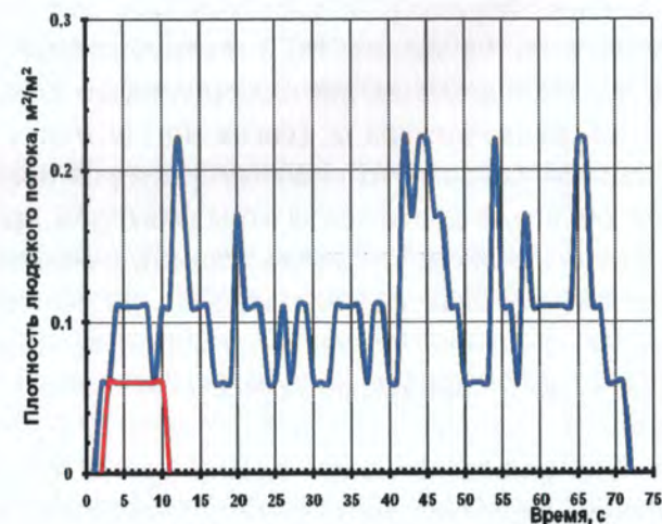
Рис. 124. Плотность людского потока на путях эвакуации (вариант 7):
