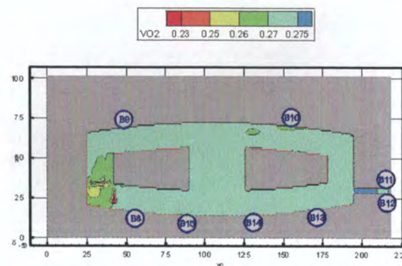
Рис. 70. Концентрация \text{O}_2 ( \text{кг}/\text{м}^3 ) в горизонтальном сечении на высоте 1,7 м от уровня пола второго этажа в момент времени 1100 с
