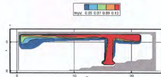
Рис. 85. Оптическая плотность дыма ( Hn/m ) в вертикальном сечении 1-1 в момент времени 130 с
