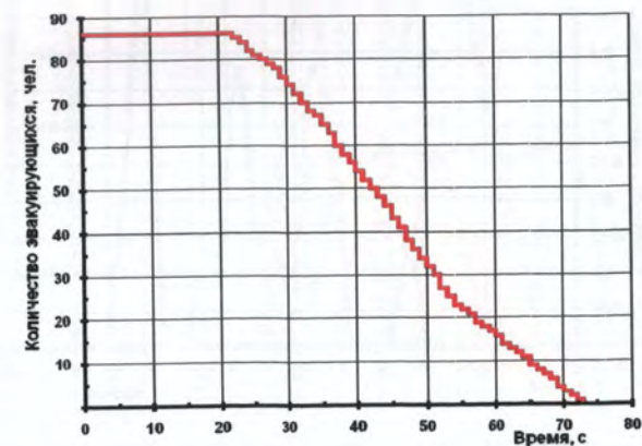
Рис. 174. Динамика эвакуации людей из здания наружу (вариант 4)
