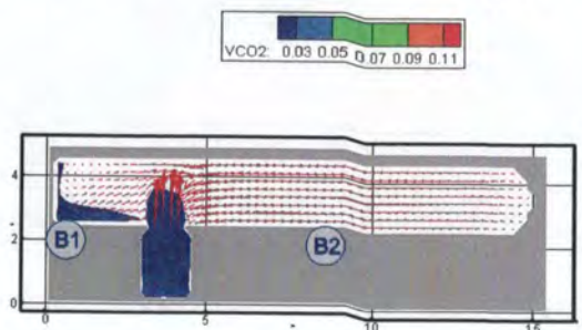
Рис. 167. Концентрация \text{CO}_2 ( \text{кг}/\text{м}^3 ) в горизонтальном сечении на высоте 1,7 м от уровня пола в момент времени 190 с
