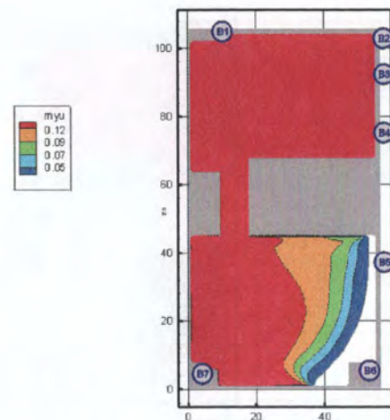
Рис. 28. Оптическая плотность дыма ( H_n/m ) в горизонтальном сечении на высоте 1,7 м от уровня пола в момент времени 300 с
