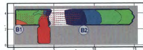
Рис. 162. Оптическая плотность дыма (Hn/м) в горизонтальном сечении на высоте 1,7 м от уровня пола в момент времени 150 с
