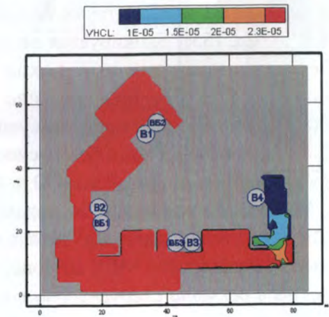
Рис. 152. Концентрация \text{HCl} ( \text{кг}/\text{м}^3 ) в горизонтальном сечении на высоте 1,7 м от уровня пола в момент времени 430 с
