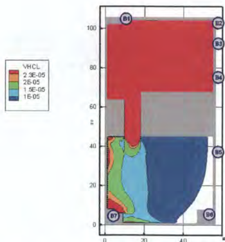
Рис. 38. Концентрация \text{HCl} ( \text{кг}/\text{м}^3 ) в горизонтальном сечении на высоте 1,7 м от уровня пола в момент времени 300 с
