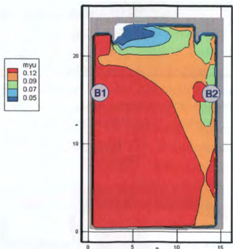
Рис. 87. Оптическая плотность дыма ( H_n/m ) в горизонтальном сечении на высоте 2,9 м от уровня пола в момент времени 230 с
