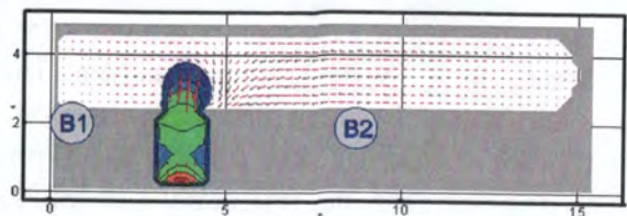
Рис. 160. Оптическая плотность дыма (Hn/м) в горизонтальном сечении на высоте 1,7 м от уровня пола в момент времени 60 с
