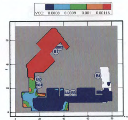
Рис. 148. Концентрация CO ( kg/m^3 ) в горизонтальном сечении на высоте 1,7 м от уровня пола в момент времени 430 с
