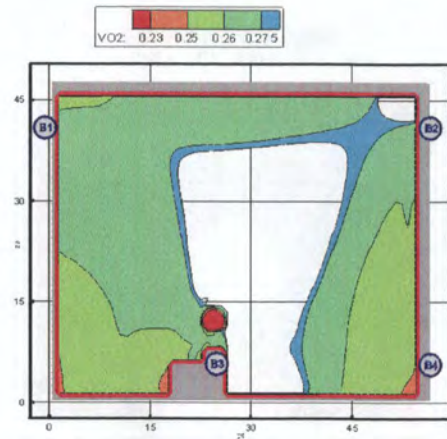
Рис. 19. Концентрация \text{O}_2 ( \text{кг}/\text{м}^3 ) в горизонтальном сечении на высоте 1,7 м от уровня пола в момент времени 100 с
