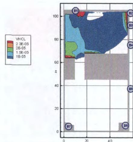
Рис. 36. Концентрация HCl ( кг/м^3 ) в горизонтальном сечении на высоте 1,7 м от уровня пола в момент времени 80 с
