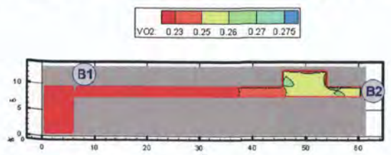
Рис. 108. Концентрация O_2 ( kg/m^3 ) в горизонтальном сечении на высоте 1,7 м от уровня пола в момент времени 290 с
