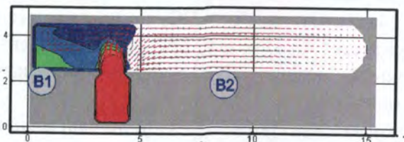
Рис. 161. Оптическая плотность дыма (Hn/м) в горизонтальном сечении на высоте 1,7 м от уровня пола в момент времени 110 с
