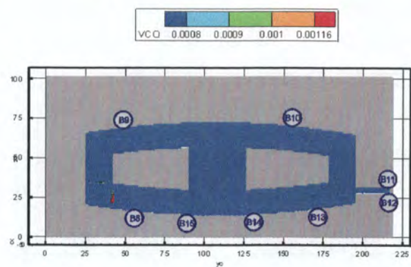
Рис. 64. Концентрация CO ( кг/м^3 ) в горизонтальном сечении на высоте 1,7 м от уровня пола второго этажа в момент времени 1100 с
