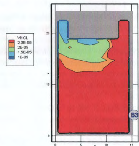
Рис. 97. Концентрация \text{HCl} ( \text{кг}/\text{м}^3 ) в горизонтальном сечении на высоте 1,7 м от уровня пола в момент времени 410 с
