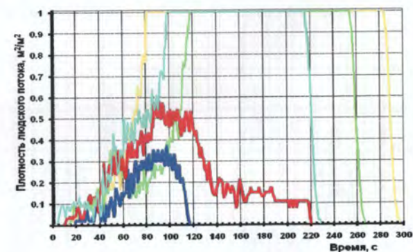
Рис. 120. Плотность людского потока на путях эвакуации (вариант 4):
