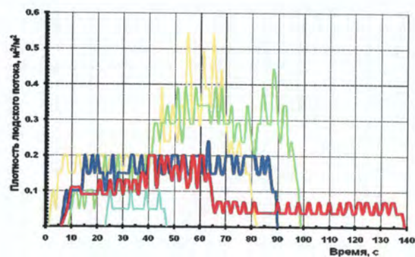
Рис. 121. Плотность людского потока на путях эвакуации (вариант 4):
