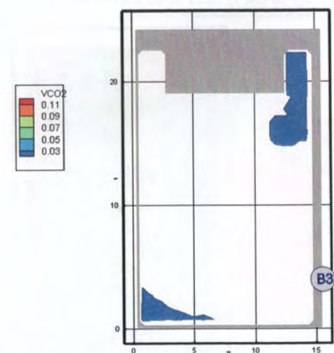
Рис. 93. Концентрация CO_2 ( kg/m^3 ) в горизонтальном сечении на высоте 1,7 м от уровня пола в момент времени 410 с
