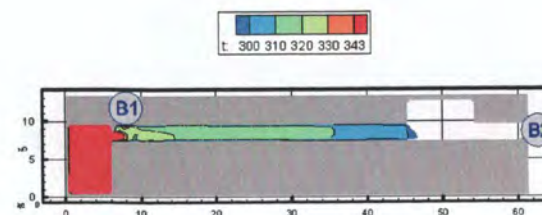
Рис. 103. Поля температуры ( K ) в горизонтальном сечении на высоте 1,7 м от уровня пола в момент времени 230 с
