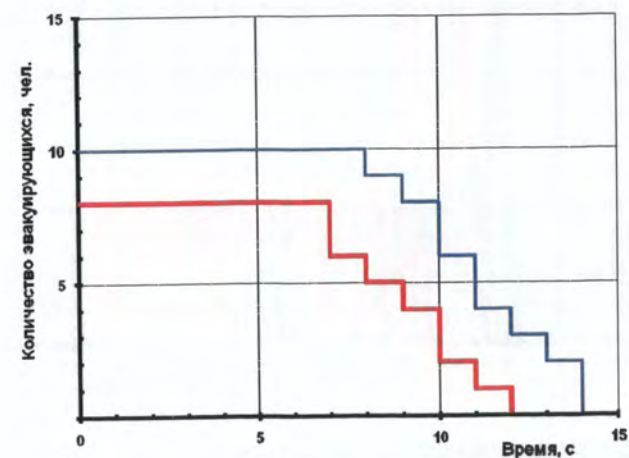
Рис. 173. Динамика эвакуации людей (вариант 4):
