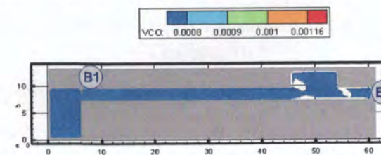
Рис. 105. Концентрация CO ( kg/m^3 ) в горизонтальном сечении на высоте 1,7 м от уровня пола в момент времени 290 с
