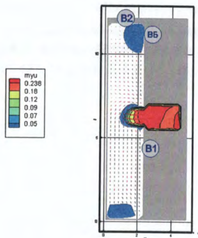
Рис. 180. Оптическая плотность дыма ( H_n/m ) в горизонтальном сечении на высоте 1,7 м от уровня пола в момент времени 100 с
