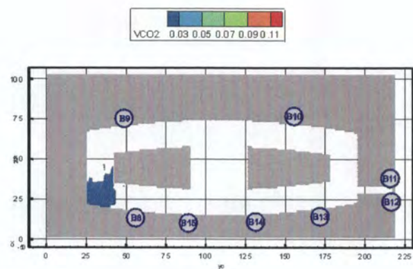
Рис. 67. Концентрация \text{CO}_2 ( \text{кг}/\text{м}^3 ) в горизонтальном сечении на высоте 1,7 м от уровня пола второго этажа в момент времени 1100 с
