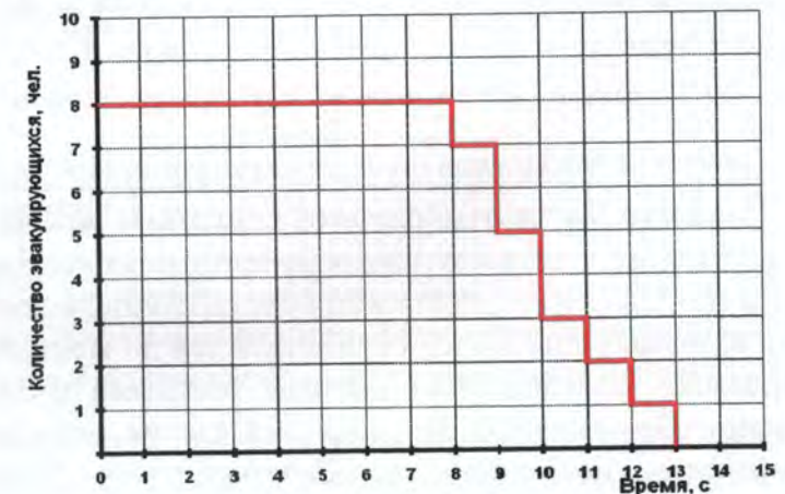
Рис. 187. Динамика эвакуации людей (вариант 5):
