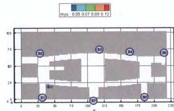
Рис. 48. Оптическая плотность дыма (Hn/м) в горизонтальном сечении на высоте 1,7 м от уровня пола первого этажа в момент времени 80 с
