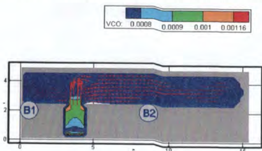
Рис. 166. Концентрация CO ( \text{кг}/\text{м}^3 ) в горизонтальном сечении на высоте 1,7 м от уровня пола в момент времени 190 с
