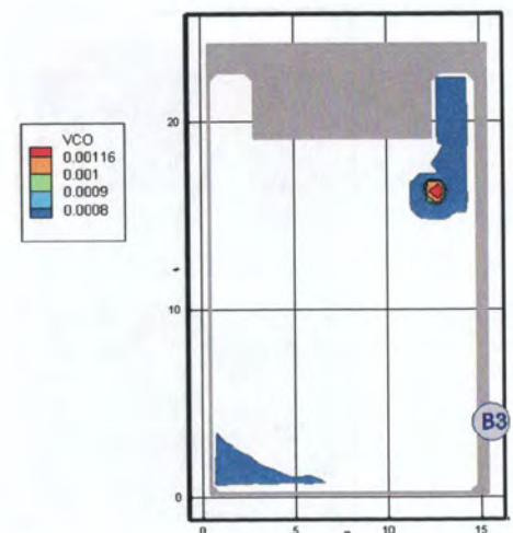
Рис. 92. Концентрация CO ( kg/m^3 ) в горизонтальном сечении на высоте 1,7 м от уровня пола в момент времени 410 с
