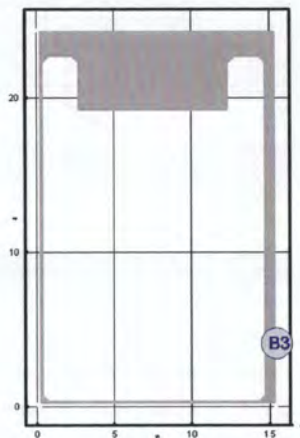
Рис. 8. Расчетная схема шестого сценария развития пожара (горизонтальное сечение на высоте 1,7 м от уровня пола):
