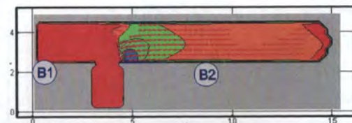
Рис. 163. Оптическая плотность дыма (Hn/м) в горизонтальном сечении на высоте 1,7 м от уровня пола в момент времени 170 с
