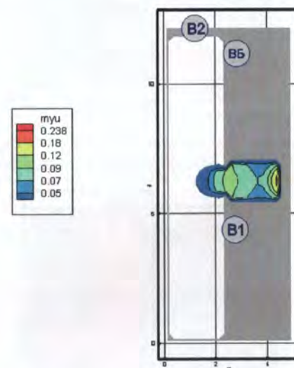
Рис. 153. Оптическая плотность дыма (Hn/м) в горизонтальном сечении на высоте 1,7 м от уровня пола в момент времени 60 с
