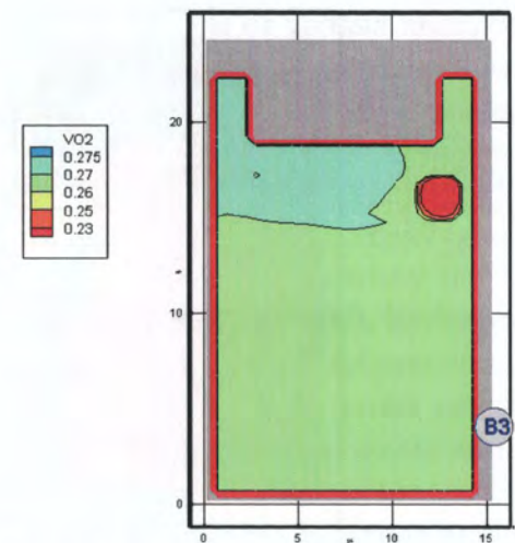
Рис. 96. Концентрация \text{O}_2 ( \text{кг}/\text{м}^3 ) в горизонтальном сечении на высоте 1,7 м от уровня пола в момент времени 410 с
