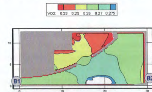
Рис. 82. Концентрация O_2 ( kg/m^3 ) в горизонтальном сечении на высоте 1,7 м от уровня пола в момент времени 220 с
