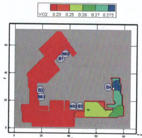
Рис. 150. Концентрация \text{O}_2 ( \text{кг}/\text{м}^3 ) в горизонтальном сечении на высоте 1,7 м от уровня пола в момент времени 430 с
