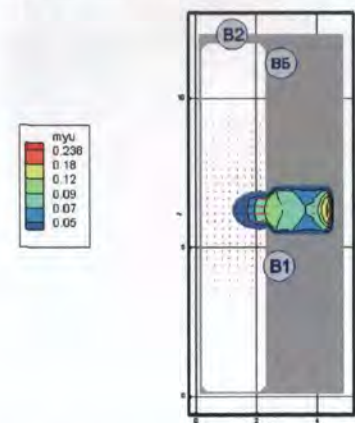
Рис. 179. Оптическая плотность дыма ( \text{Hn}/\text{м} ) в горизонтальном сечении на высоте 1,7 м от уровня пола в момент времени 60 с
