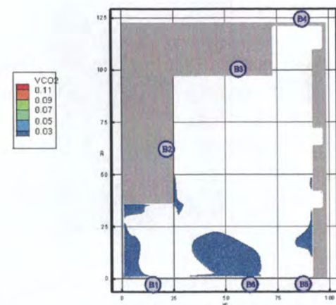
Рис. 45. Концентрация CO 2 ( \text{кг/м}^3 ) в горизонтальном сечении на высоте 1,7 м от уровня пола в момент времени 1100 с
