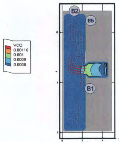
Рис. 184. Концентрация CO ( кг/м^3 ) в горизонтальном сечении на высоте 1,7 м от уровня пола в момент времени 180 с
