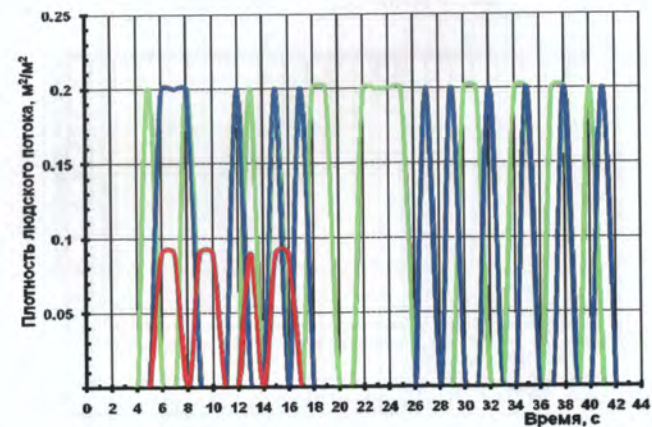
Рис. 116. Плотность людского потока на путях эвакуации (вариант 1):
