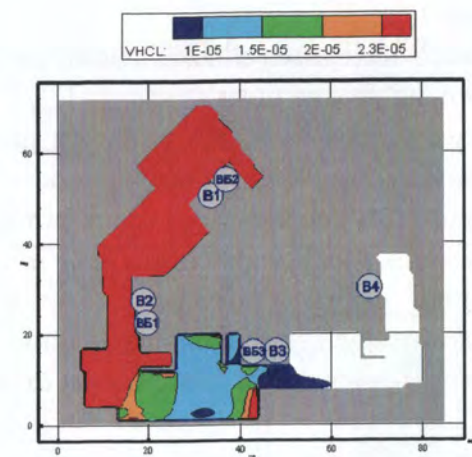
Рис. 151. Концентрация \text{HCl} ( \text{кг}/\text{м}^3 ) в горизонтальном сечении на высоте 1,7 м от уровня пола в момент времени 260 с
