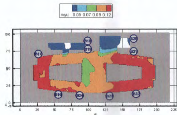
Рис. 56. Оптическая плотность дыма ( H_n/m ) в горизонтальном сечении на высоте 1,7 м от уровня пола третьего этажа в момент времени 900 с
