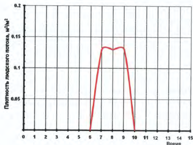
Рис. 188. Плотность людского потока на путях эвакуации (вариант 5): — перед выходом В1
