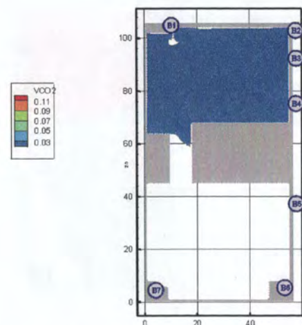
Рис. 32. Концентрация \text{CO}_2 ( \text{кг/м}^3 ) в горизонтальном сечении на высоте 1,7 м от уровня пола в момент времени 300 с
