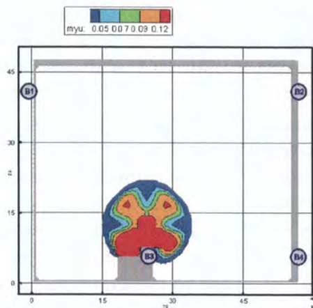
Рис. 11. Оптическая плотность дыма ( \text{Hn/m} ) в горизонтальном сечении на высоте 1,7 м от уровня пола в момент времени 20 с
