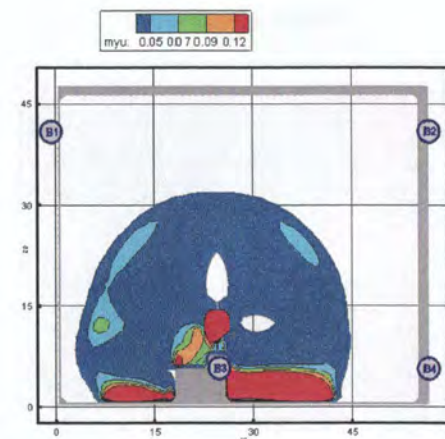
Рис. 12. Оптическая плотность дыма ( \text{Hn/m} ) в горизонтальном сечении на высоте 1,7 м от уровня пола в момент времени 40 с
