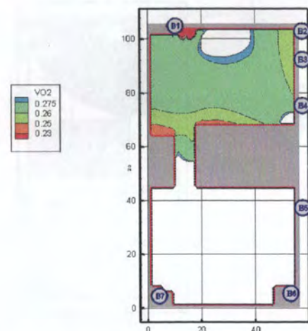
Рис. 33. Концентрация \text{O}_2 ( \text{кг/м}^3 ) в горизонтальном сечении на высоте 1,7 м от уровня пола в момент времени 100 с
