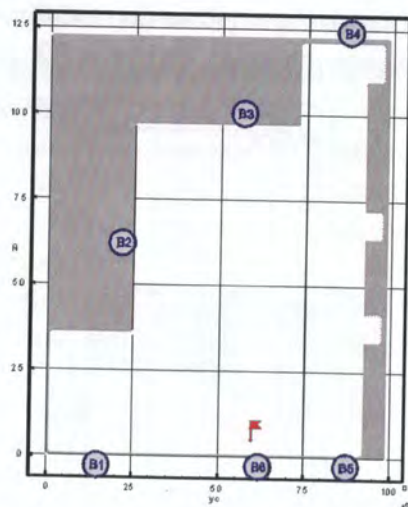
Рис. 3. Расчетная схема третьего сценария развития пожара (горизонтальное сечение на высоте 1,7 м от уровня пола): B1–B5 – эвакуационные выходы
