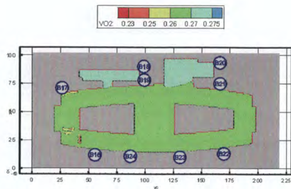
Рис. 71. Концентрация O_2 ( кг/м^3 ) в горизонтальном сечении на высоте 1,7 м от уровня пола третьего этажа в момент времени 1100 с
