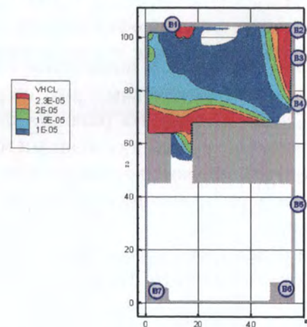
Рис. 37. Концентрация HCl ( кг/м^3 ) в горизонтальном сечении на высоте 1,7 м от уровня пола в момент времени 100 с
