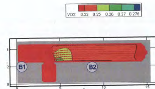
Рис. 168. Концентрация \text{O}_2 ( \text{кг}/\text{м}^3 ) в горизонтальном сечении на высоте 1,7 м от уровня пола в момент времени 190 с
