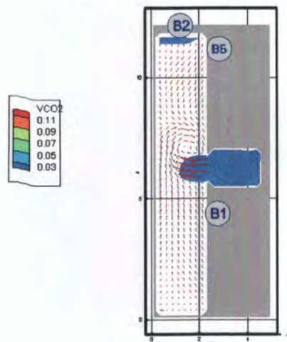
Рис. 185. Концентрация CO_2 ( кг/м^3 ) в горизонтальном сечении на высоте 1,7 м от уровня пола в момент времени 180 с
