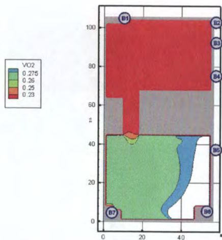
Рис. 34. Концентрация O_2 ( кг/м^3 ) в горизонтальном сечении на высоте 1,7 м от уровня пола в момент времени 300 с
