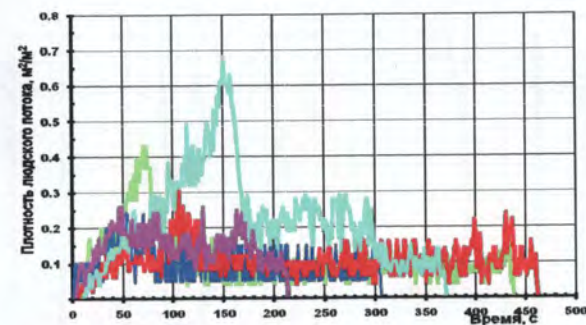
Рис. 119. Плотность людского потока на путях эвакуации (вариант 4):
