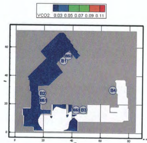
Рис. 149. Концентрация \text{CO}_2 ( \text{кг}/\text{м}^3 ) в горизонтальном сечении на высоте 1,7 м от уровня пола в момент времени 430 с
