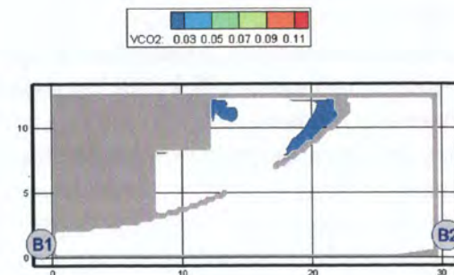
Рис. 81. Концентрация CO_2 ( kg/m^3 ) в горизонтальном сечении на высоте 1,7 м от уровня пола в момент времени 220 с
