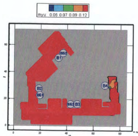
Рис. 145. Оптическая плотность дыма ( H_n/m ) в горизонтальном сечении на высоте 1,7 м от уровня пола в момент времени 430 с
