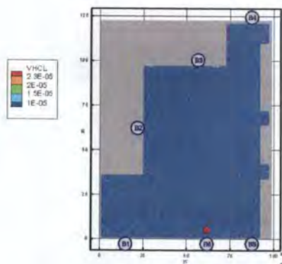
Рис. 47. Концентрация HCl ( кг/м^3 ) в горизонтальном сечении на высоте 1,7 м от уровня пола в момент времени 1100 с
