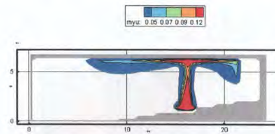
Рис. 84. Оптическая плотность дыма ( Hn/m ) в вертикальном сечении 1-1 в момент времени 80 с
