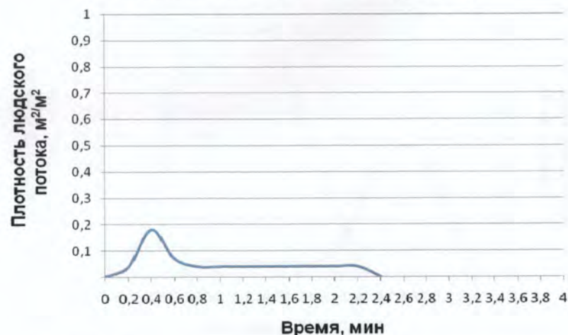
Рис. 194. Зависимость плотности людского потока от времени на лестничной площадке на уровне 3-го этажа
