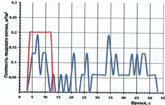
Рис. 122. Плотность людского потока на путях эвакуации (вариант 5):
