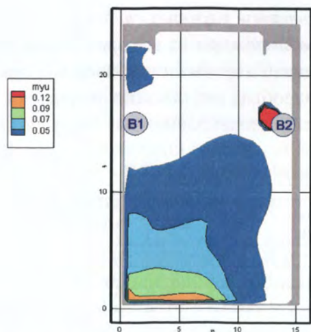
Рис. 86. Оптическая плотность дыма ( H_n/m ) в горизонтальном сечении на высоте 2,9 м от уровня пола в момент времени 170 с
