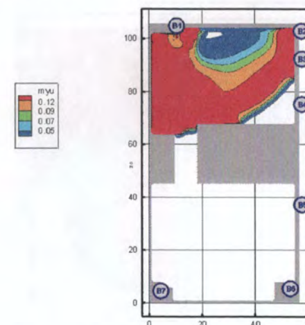
Рис. 25. Оптическая плотность дыма ( H_n/m ) в горизонтальном сечении на высоте 1,7 м от уровня пола в момент времени 80 с
