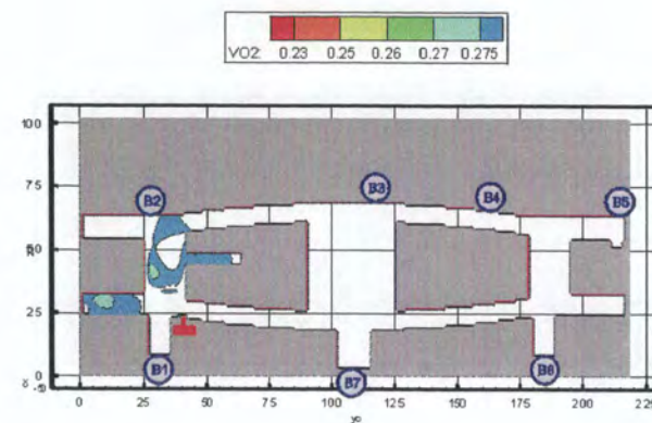
Рис. 69. Концентрация \text{O}_2 ( \text{кг}/\text{м}^3 ) в горизонтальном сечении на высоте 1,7 м от уровня пола первого этажа в момент времени 1100 с
