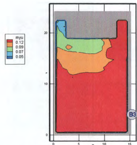
Рис. 88. Оптическая плотность дыма ( H_n/m ) в горизонтальном сечении на высоте 1,7 м от уровня пола в момент времени 410 с
