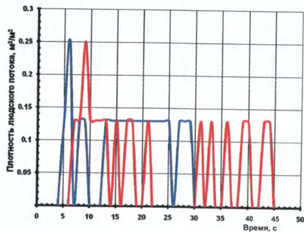
Рис. 175. Плотность людского потока на путях эвакуации (вариант 1): — перед выходом B3; — перед выходом B2
