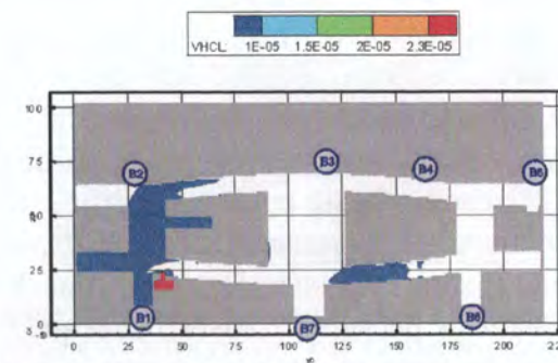
Рис. 74. Концентрация HCl ( кг/м^3 ) в горизонтальном сечении на высоте 1,7 м от уровня пола первого этажа в момент времени 1100 с
