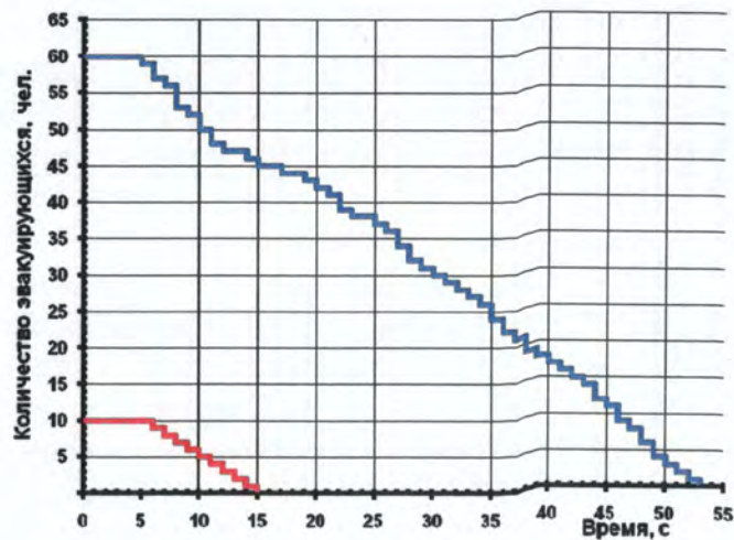
Рис. 113. Динамика эвакуации людей (вариант 5):
