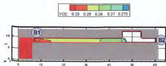
Рис. 107. Концентрация O_2 ( kg/m^3 ) в горизонтальном сечении на высоте 1,7 м от уровня пола в момент времени 230 с
