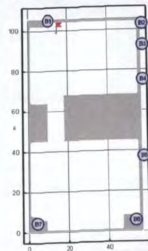
Рис. 2. Расчетная схема второго сценария развития пожара (горизонтальное сечение на высоте 1,7 м от уровня пола): В1–В7 – эвакуационные выходы
