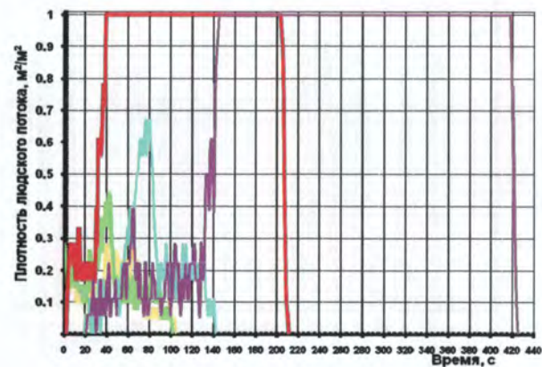
Рис. 118. Плотность людского потока на путях эвакуации (вариант 3):
