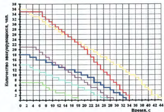
Рис. 111. Динамика эвакуации людей (вариант 2):
