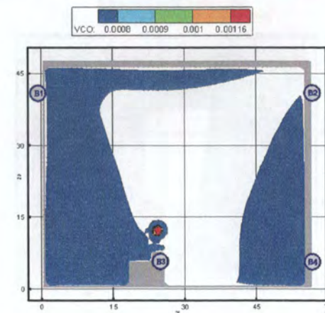
Рис. 17. Концентрация CO ( kg/m^3 ) в горизонтальном сечении на высоте 1,7 м от уровня пола в момент времени 100 с
