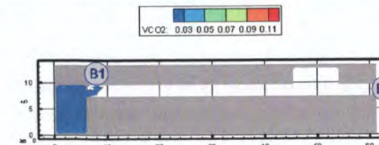
Рис. 106. Концентрация CO_2 ( kg/m^3 ) в горизонтальном сечении на высоте 1,7 м от уровня пола в момент времени 290 с
