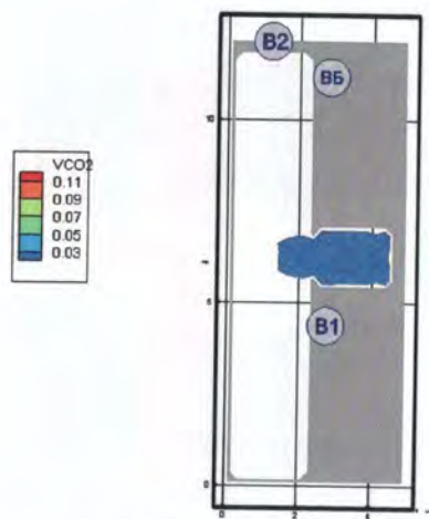
Рис. 158. Концентрация CO_2 ( кг/м^3 ) в горизонтальном сечении на высоте 1,7 м от уровня пола в момент времени 160 с
