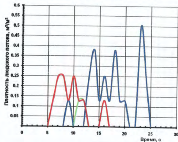
Рис. 176. Плотность людского потока на путях эвакуации (вариант 2): — перед выходом B1; — перед выходом B3; — перед выходом B4
