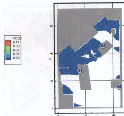
Рис. 136. Концентрация CO_2 ( kg/m^3 ) в горизонтальном сечении на высоте 1,7 м от уровня пола в момент времени 200 с
