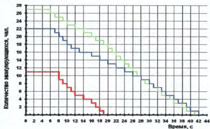
Рис. 110. Динамика эвакуации людей (вариант 1):
