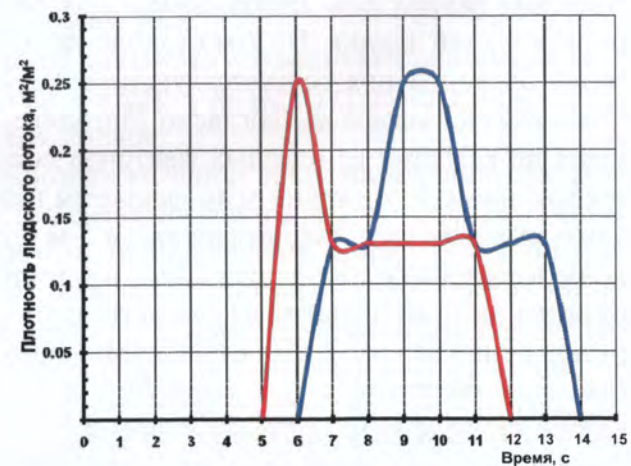
Рис. 178. Плотность людского потока на путях эвакуации (вариант 4): — перед выходом B1; — перед выходом B2
