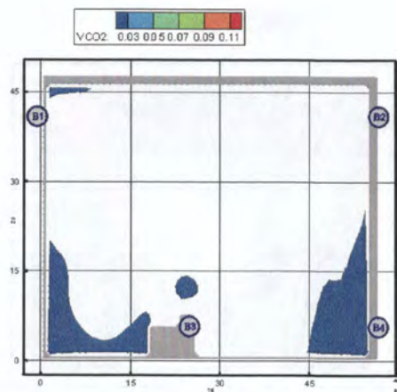
Рис. 18. Концентрация \text{CO}_2 ( \text{кг}/\text{м}^3 ) в горизонтальном сечении на высоте 1,7 м от уровня пола в момент времени 100 с
