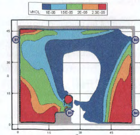
Рис. 21. Концентрация \text{HCl} ( \text{кг}/\text{м}^3 ) в горизонтальном сечении на высоте 1,7 м от уровня пола в момент времени 100 с
