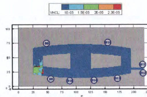
Рис. 73. Концентрация HCl ( кг/м^3 ) в горизонтальном сечении на высоте 1,7 м от уровня пола второго этажа в момент времени 1100 с
