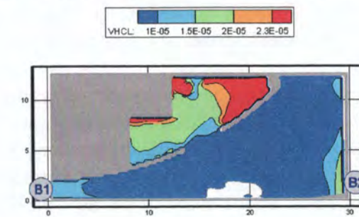
Рис. 83. Концентрация HCl ( kg/m^3 ) в горизонтальном сечении на высоте 1,7 м от уровня пола в момент времени 220 с
