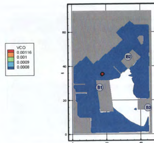
Рис. 135. Концентрация CO ( kg/m^3 ) в горизонтальном сечении на высоте 1,7 м от уровня пола в момент времени 200 с
