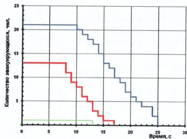
Рис. 171. Динамика эвакуации людей (вариант 2):
