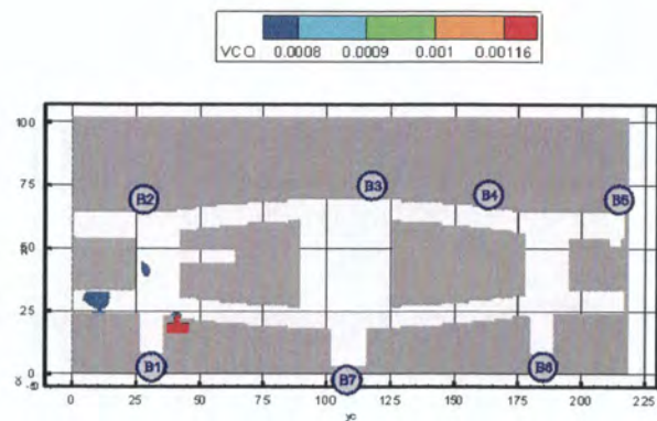
Рис. 63. Концентрация CO ( кг/м^3 ) в горизонтальном сечении на высоте 1,7 м от уровня пола первого этажа в момент времени 1100 с
