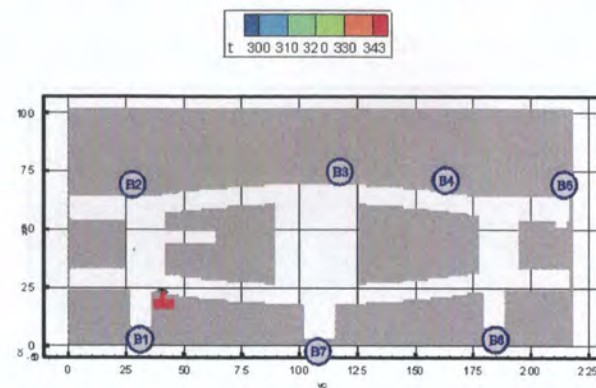
Рис. 62. Поля температуры (K) в горизонтальном сечении на высоте 1,7 м от уровня пола первого этажа в момент времени 1100 с
