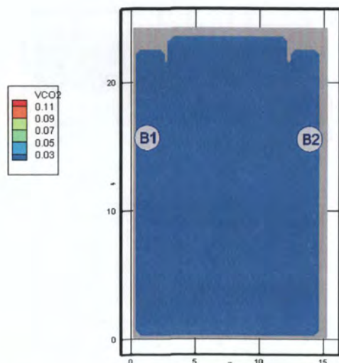
Рис. 94. Концентрация \text{CO}_2 ( \text{кг}/\text{м}^3 ) в горизонтальном сечении на высоте 2,9 м от уровня пола в момент времени 410 с
