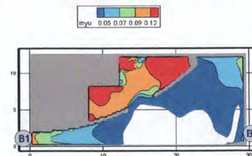
Рис. 77. Оптическая плотность дыма (Hn/m) в горизонтальном сечении на высоте 1,7 м от уровня пола в момент времени 200 с
