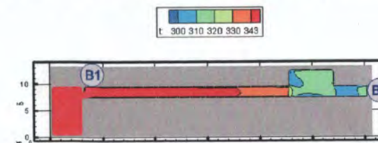
Рис. 104. Поля температуры ( K ) в горизонтальном сечении на высоте 1,7 м от уровня пола в момент времени 290 с
