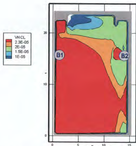
Рис. 98. Концентрация \text{HCl} ( \text{кг}/\text{м}^3 ) в горизонтальном сечении на высоте 1,7 м от уровня пола в момент времени 230 с
