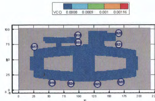
Рис. 65. Концентрация CO ( кг/м^3 ) в горизонтальном сечении на высоте 1,7 м от уровня пола третьего этажа в момент времени 1100 с
