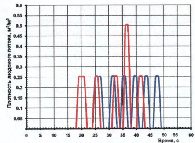
Рис. 177. Плотность людского потока на путях эвакуации (вариант 3): — перед выходом B1; — перед выходом B2
