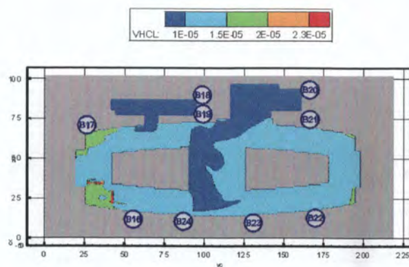
Рис. 72. Концентрация HCl ( кг/м^3 ) в горизонтальном сечении на высоте 1,7 м от уровня пола третьего этажа в момент времени 1100 с
