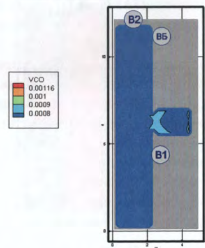
Рис. 157. Концентрация CO ( кг/м^3 ) в горизонтальном сечении на высоте 1,7 м от уровня пола в момент времени 160 с
