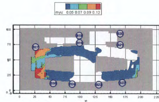
Рис. 53. Оптическая плотность дыма ( H_n/m ) в горизонтальном сечении на высоте 1,7 м от уровня пола третьего этажа в момент времени 600 с
