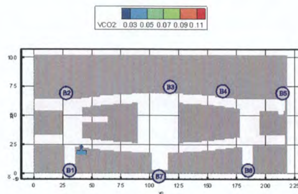
Рис. 68. Концентрация \text{CO}_2 ( \text{кг}/\text{м}^3 ) в горизонтальном сечении на высоте 1,7 м от уровня пола первого этажа в момент времени 1100 с
