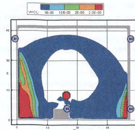
Рис. 20. Концентрация \text{HCl} ( \text{кг}/\text{м}^3 ) в горизонтальном сечении на высоте 1,7 м от уровня пола в момент времени 70 с
