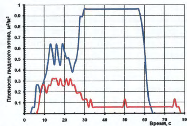
Рис. 123. Плотность людского потока на путях эвакуации (вариант 6):
