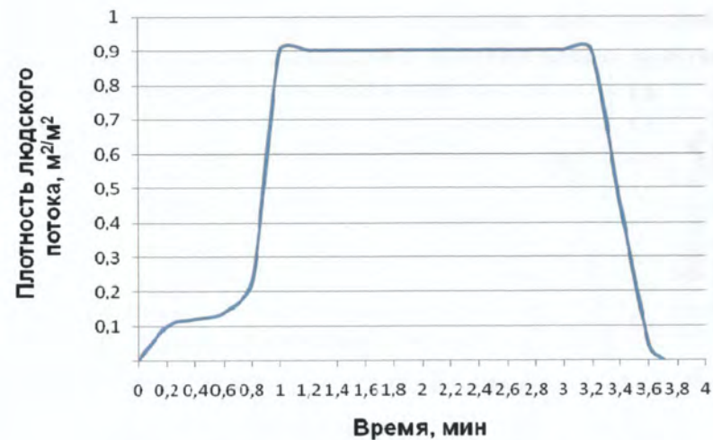
Рис. 197. Зависимость плотности людского потока от времени на выходе из здания (выход 1)
