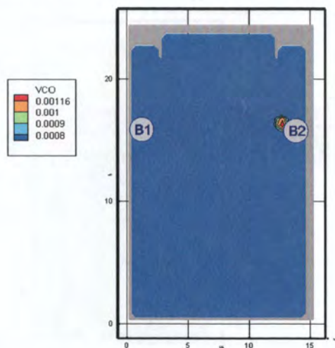
Рис. 91. Концентрация CO ( kg/m^3 ) в горизонтальном сечении на высоте 2,9 м от уровня пола в момент времени 410 с
