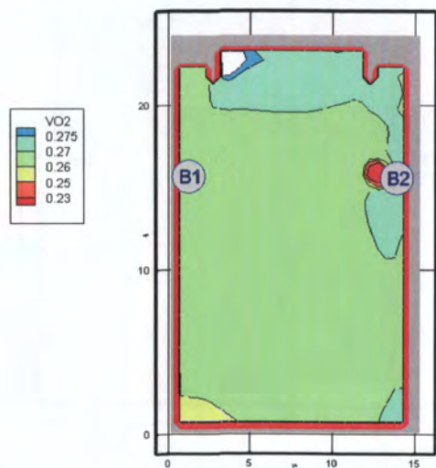
Рис. 95. Концентрация \text{O}_2 ( \text{кг}/\text{м}^3 ) в горизонтальном сечении на высоте 2,9 м от уровня пола в момент времени 230 с
