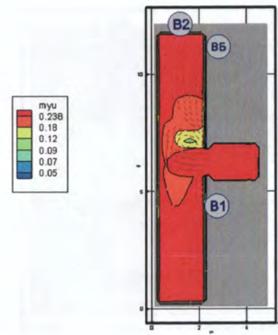
Рис. 182. Оптическая плотность дыма ( H_n/m ) в горизонтальном сечении на высоте 1,7 м от уровня пола в момент времени 180 с
