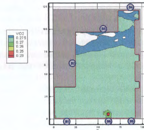
Рис. 46. Концентрация O 2 ( \text{кг/м}^3 ) в горизонтальном сечении на высоте 1,7 м от уровня пола в момент времени 1100 с
